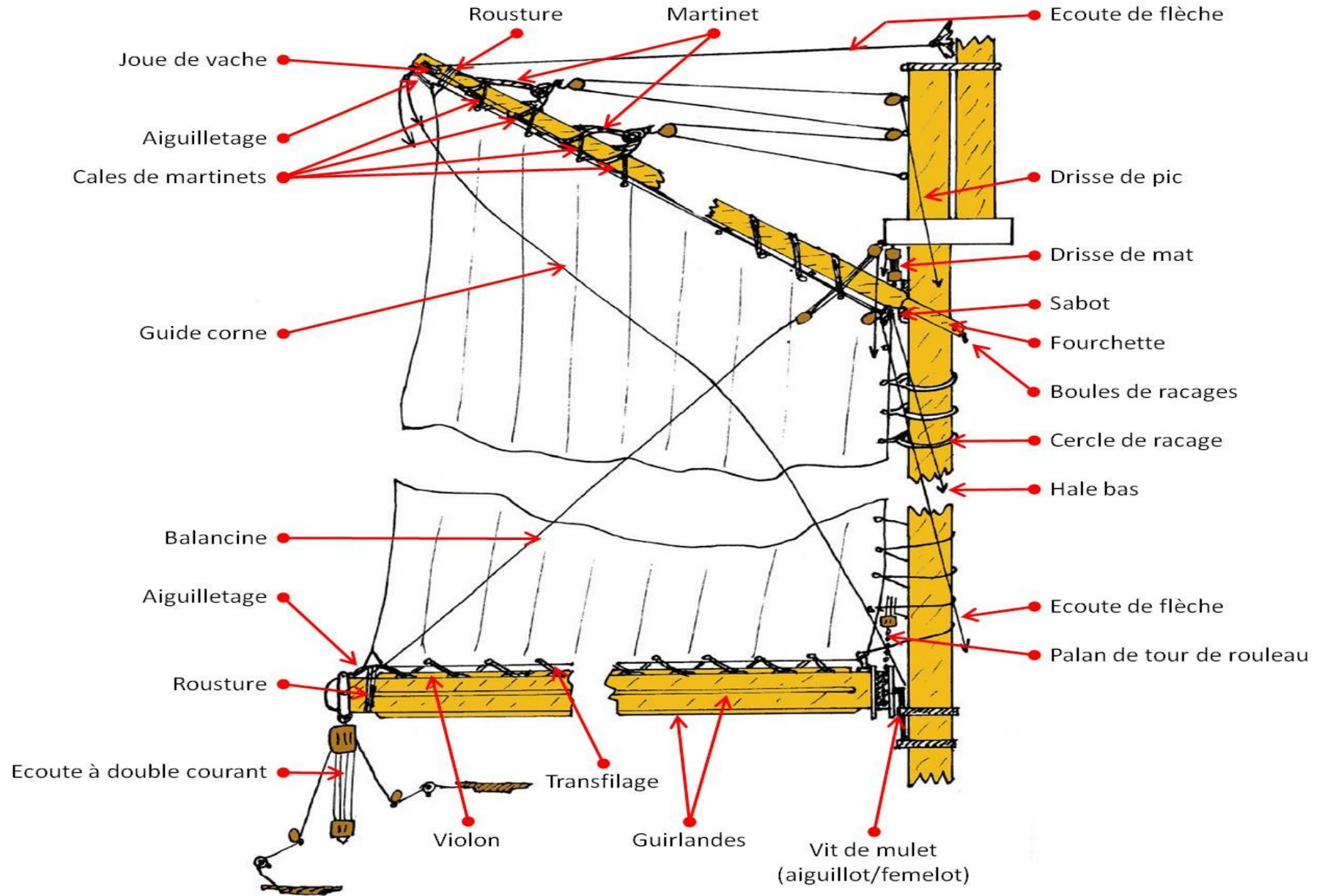
Schéma 9 : Grand'voile
