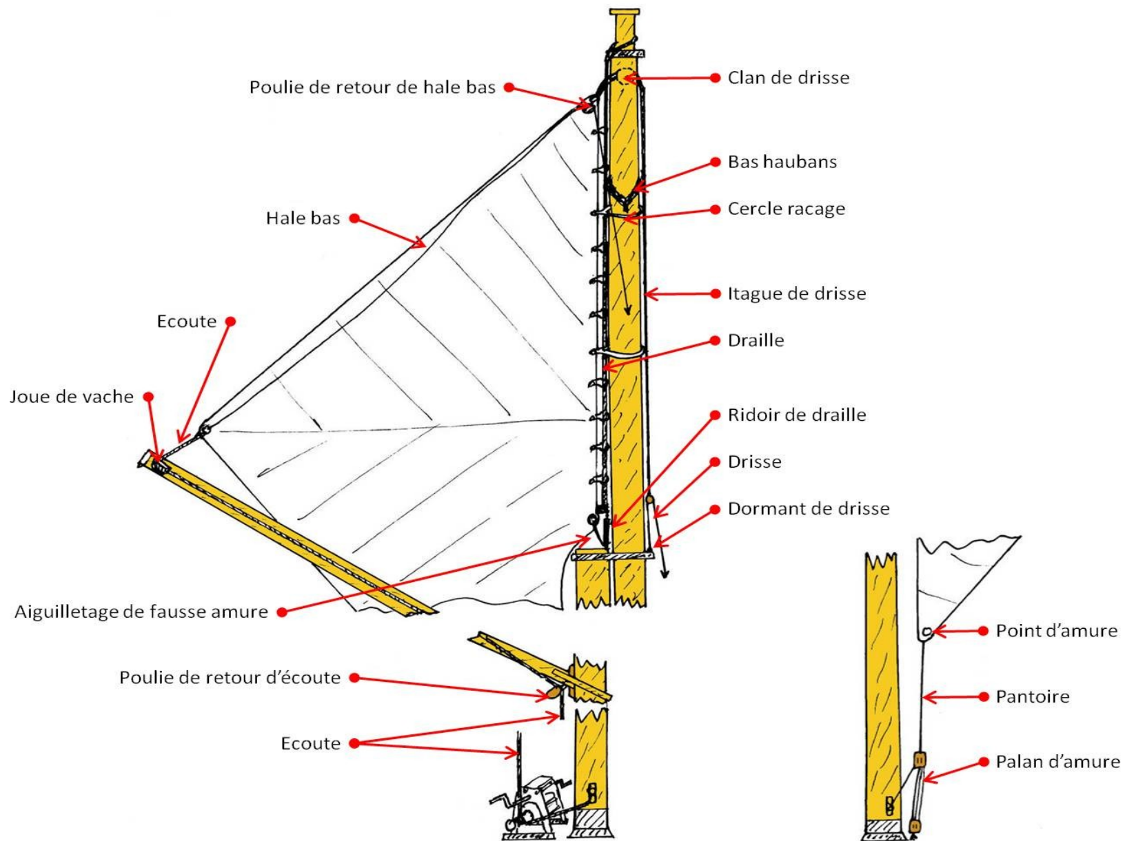
Schéma 12 : Gréement du flèche Copyright®matter-roussel-jolivet Marine Nationale - 2011
