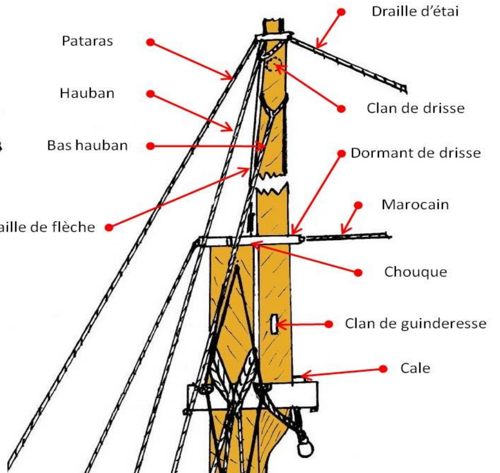
Schéma 11 : Gréement dormant en tête du mât de flèche
